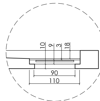
DETALLE A: hueco rejilla/sifón
