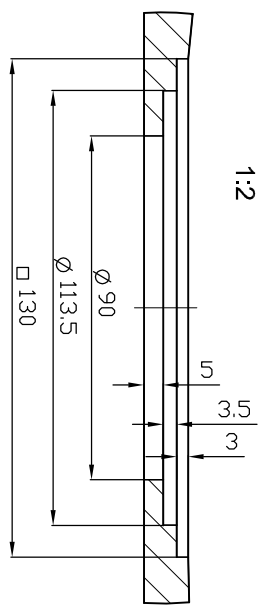
DETALLE Hueco sifón - V
