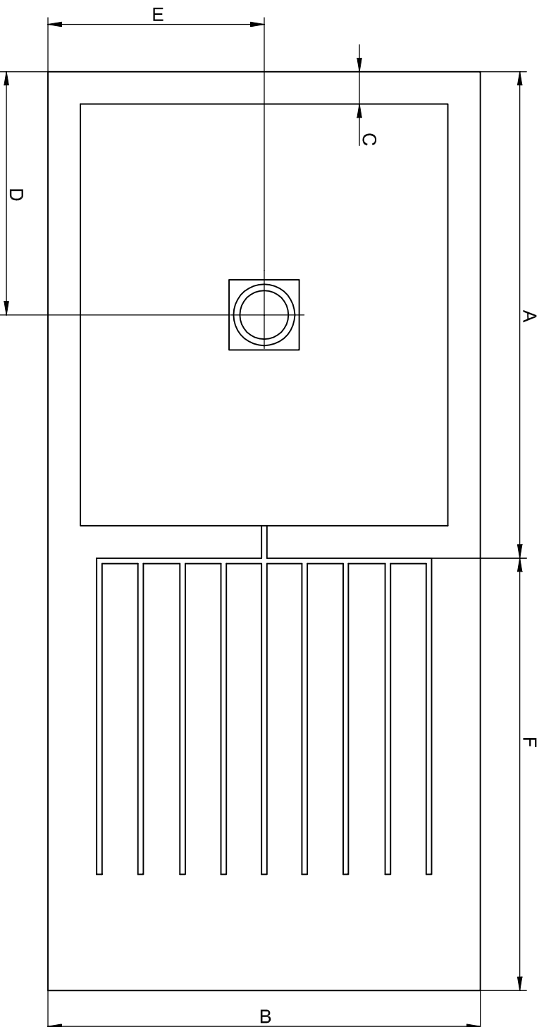
DETALLE Hueco sifón - V
