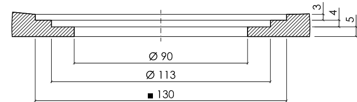
Detalle hueco sifón - V/ Shower trap hole detail - V E:1/5 / S:1/5
