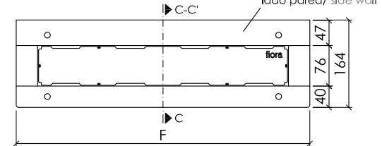
PLANTA / TOP VIEW
